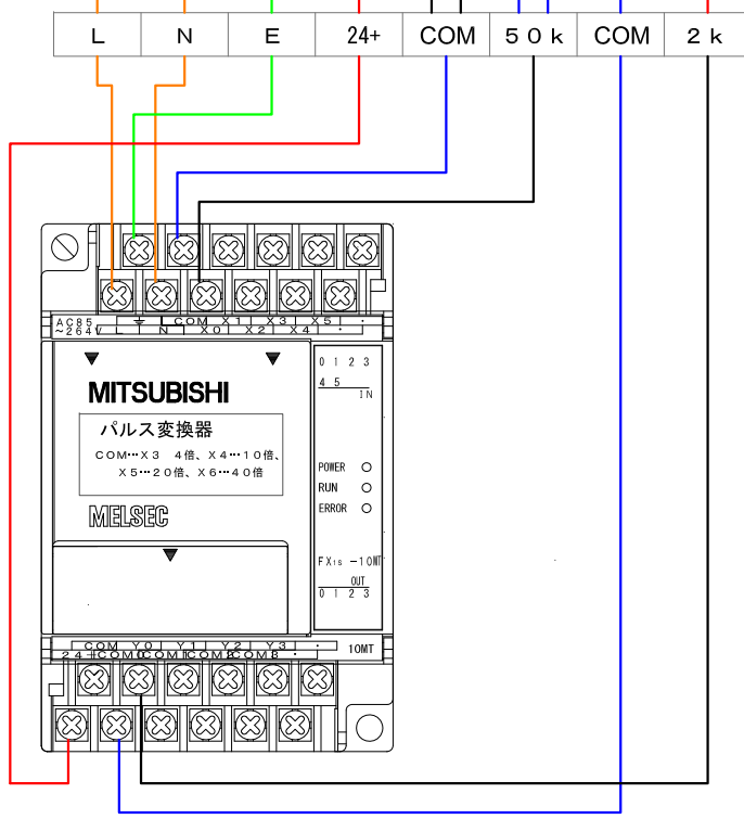
パルス変換器 IW-5(1S)
